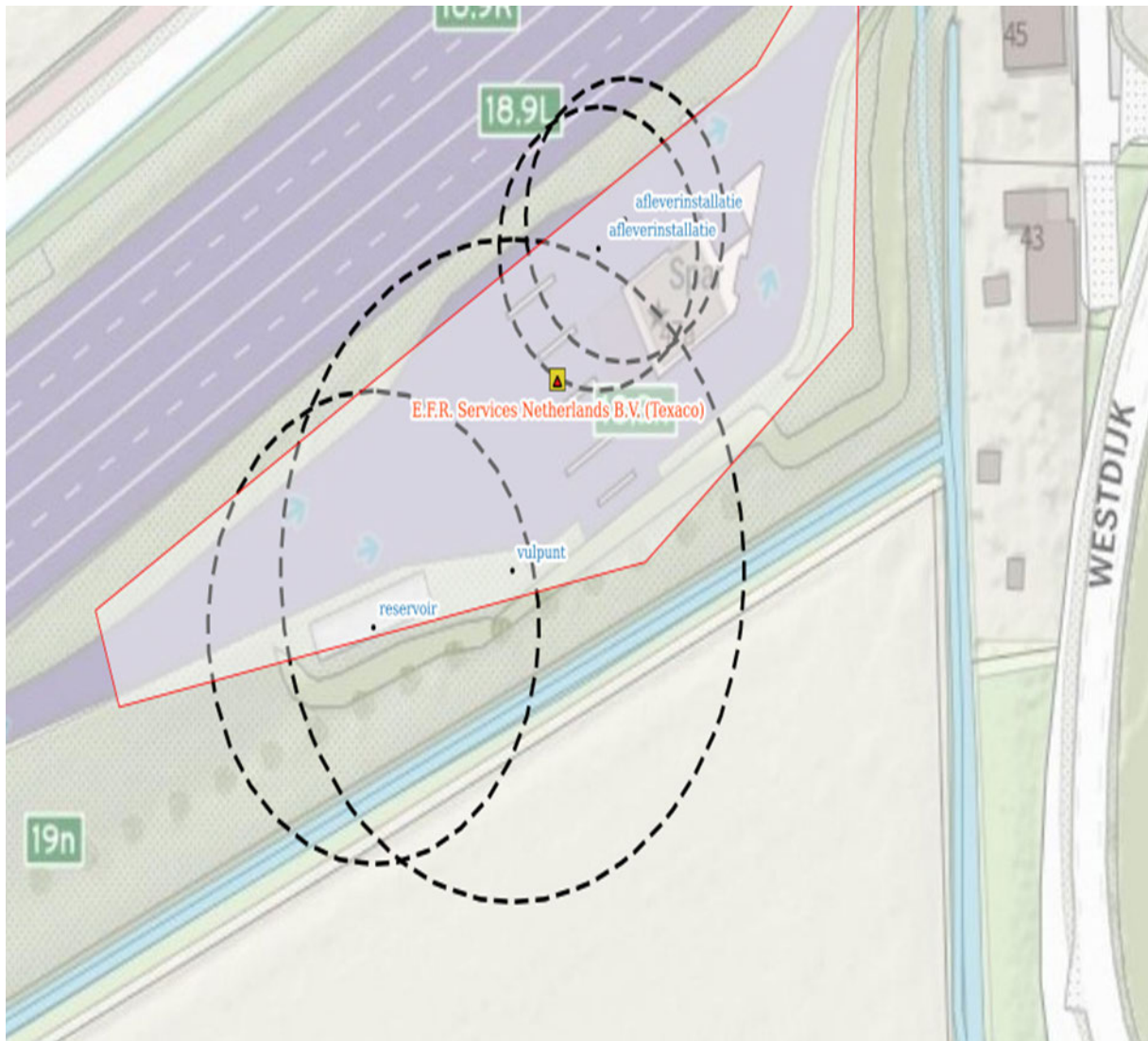
Afbeelding 1: PR 10^{-6} /jr. risicocontouren vulpunt, reservoir en afleverzuil Esso Rijksweg A29, (bron: Register Risicosituaties Gevaarlijke Stoffen).
