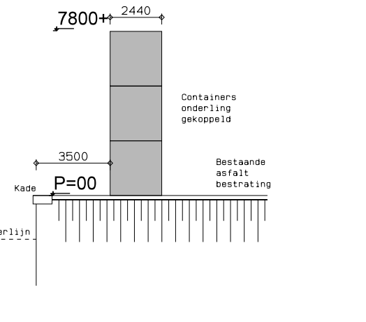
Doorsnede GS-5 tpv 3-hoog
