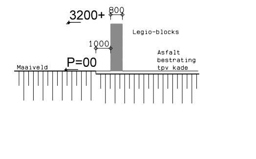
Doorsnede GS-6
