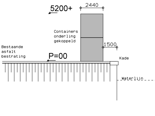
Doorsnede GS-5 tpv 2-hoog
