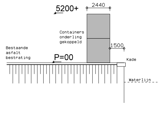
Doorsnede GS-3
