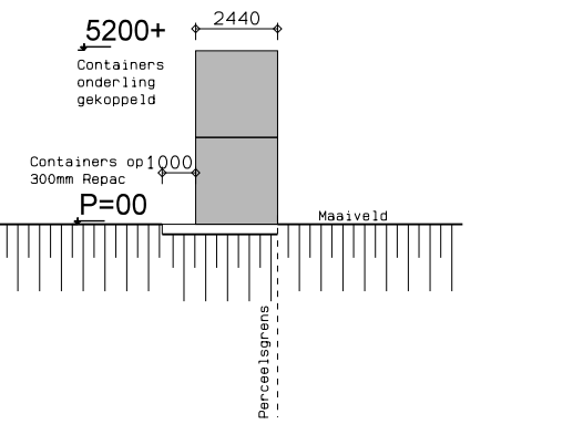
Doorsnede GS-7
