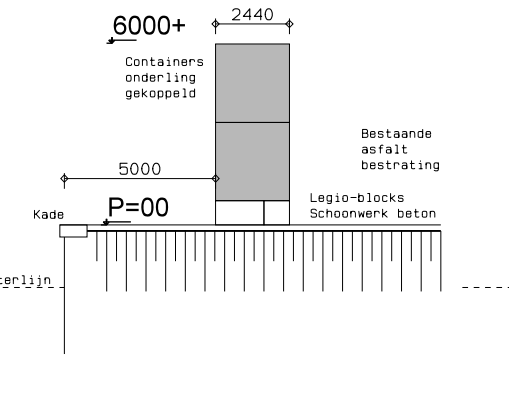
Doorsnede GS-4
