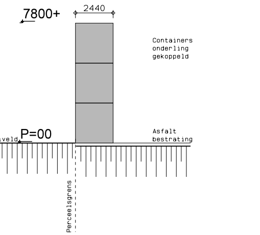
Doorsnede GS-8
