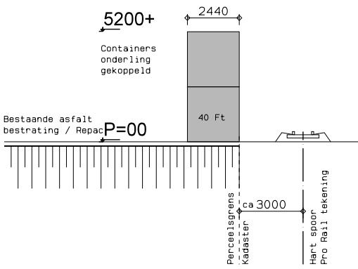
Doorsnede GS-1
