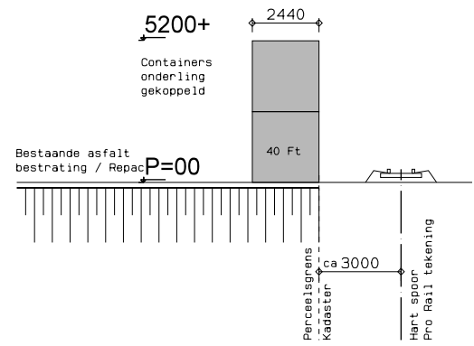
Doorsnede GS-2
