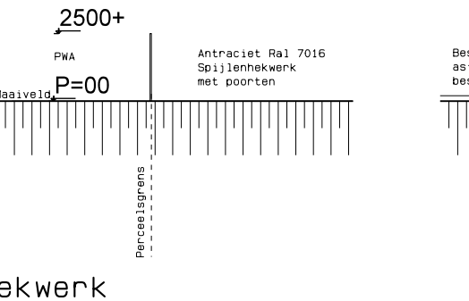
Doorsnede GS-10
