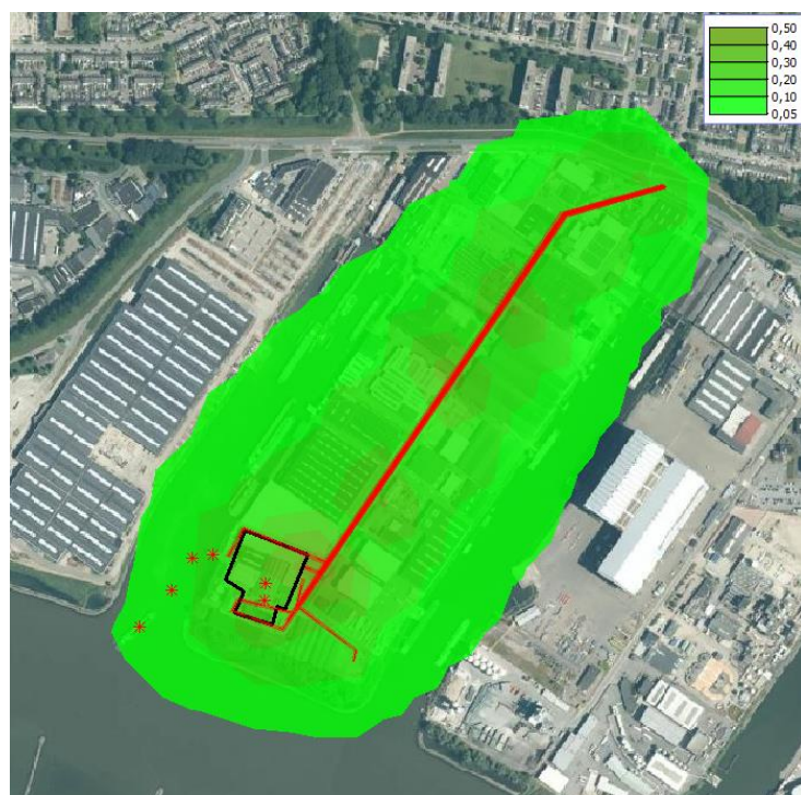
Figuur 4-1 Contour van de \text{NO}_x -bijdrage
