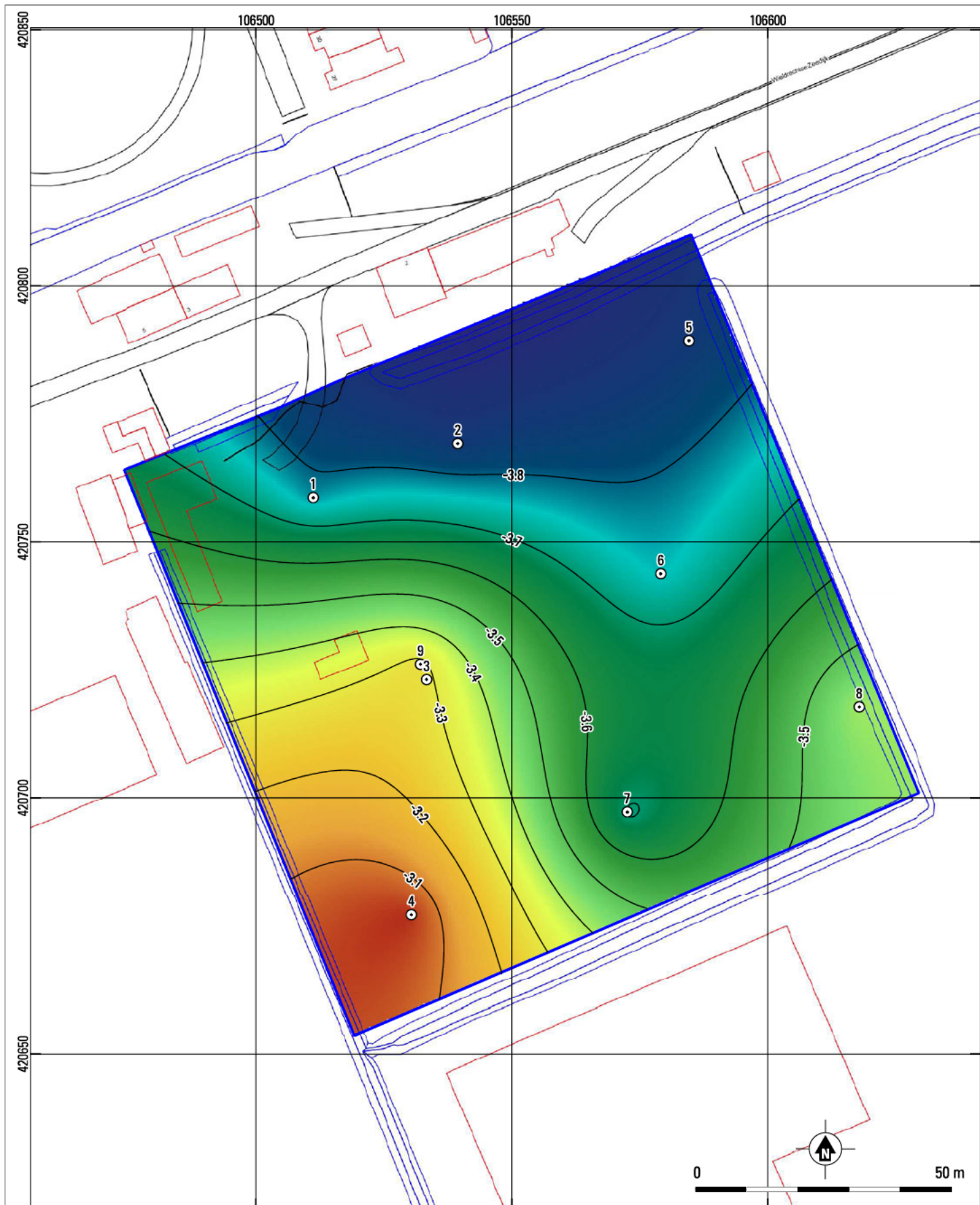
Bijlage 6. Dordrecht - Wieldrechtse Zeedijk 2a. Top van het Hollandveen in m NAP
