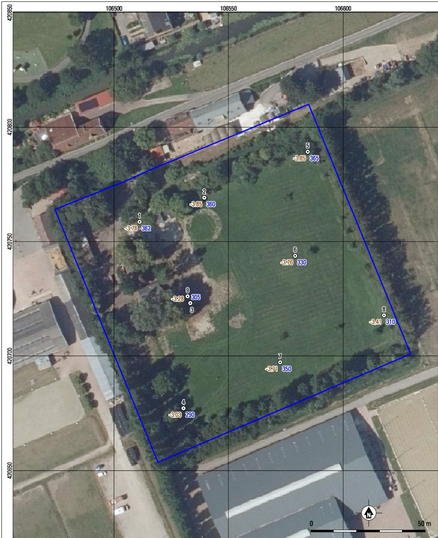
Bijlage 4. Dordrecht - Wieldrechtse Zeedijk 2a. Boorpunten op de meest recente luchtfoto.
