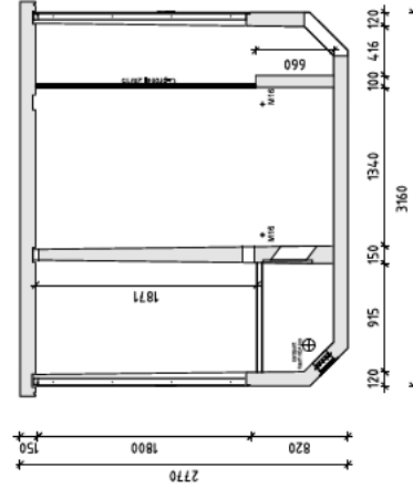
DOORSNEDE C-C
