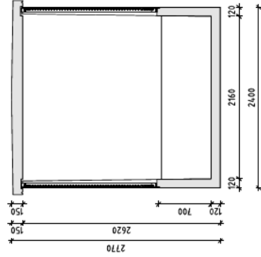
DOORSNEDE B-B
