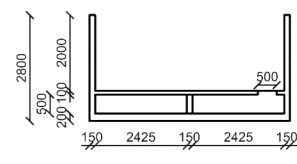
DOORSNEDEN: C-C vaste mestopslag Voorbeeld: 1:100 Aanpak: 1:100 Aanpak: 1:100 Aanpak: 1:100
